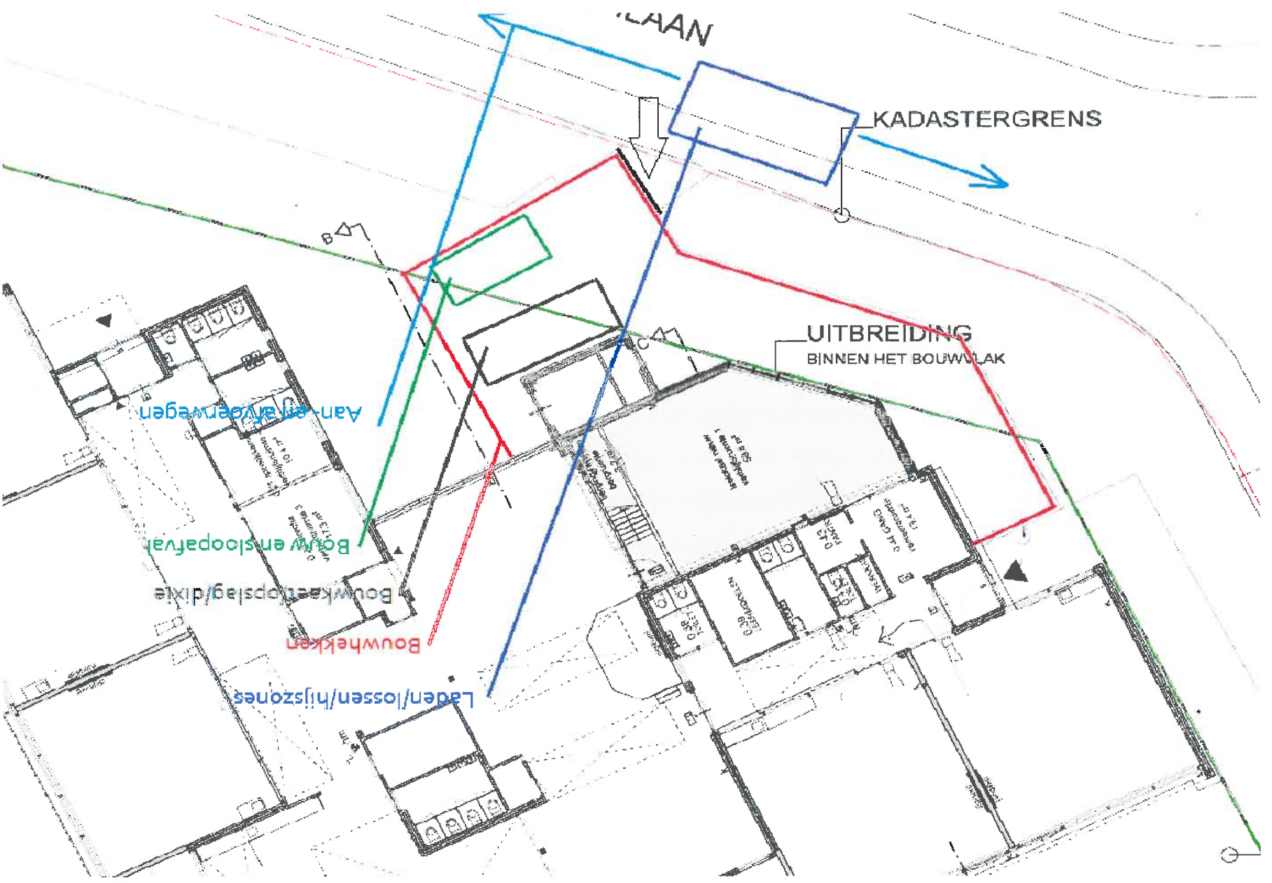
concept bouwplaatsinrichting Montessorischool 04-05-2018
